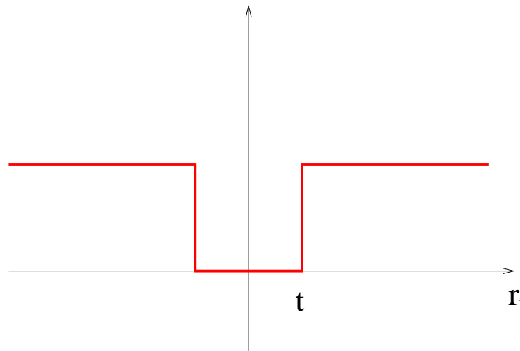
Fig. 21. RANSAC loss function
